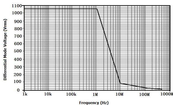
图 2 DP6150B 最大差模电压 VS 频率
