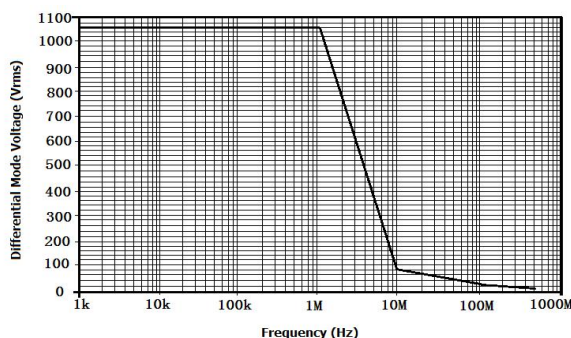
图 2 DP6150D 最大差模电压 VS 频率
