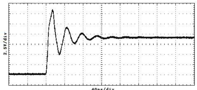
添加输入延长线(CK-301)的波形
