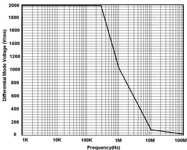
图 3: DP6280D 最大差模电压 VS 频率
